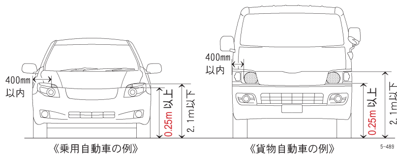
▪ 車幅灯の取付位置
